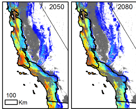
Warmer drier
