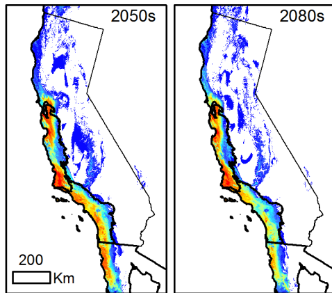
Warmer drier
