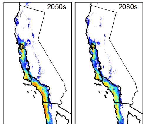
Warmer drier
