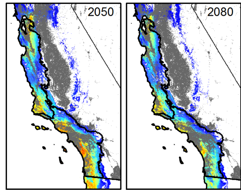
Warmer drier
