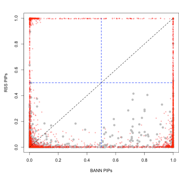
(D) SNP-Set Methods (Polygenic Traits)
