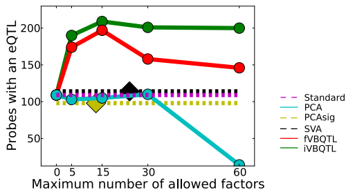
(d) Downstream (trans) eQTLs (permutation test)
