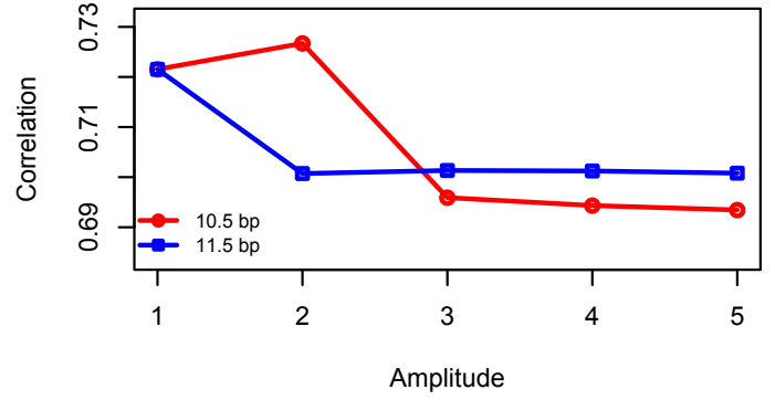
cMyc-E2f1
