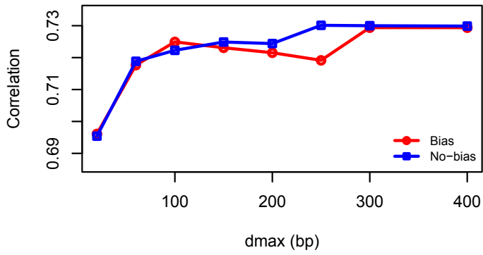
cMyc-E2f1
