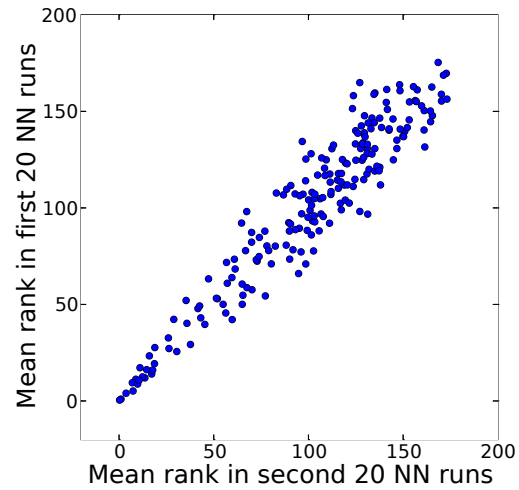
(b) ANN Reproducibility
